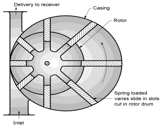
Fig. 5.9 Vane Blower
