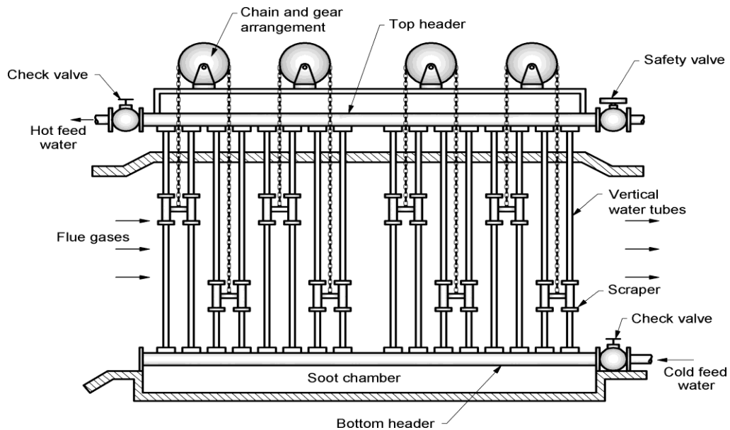
Fig. 2.12 Economiser
