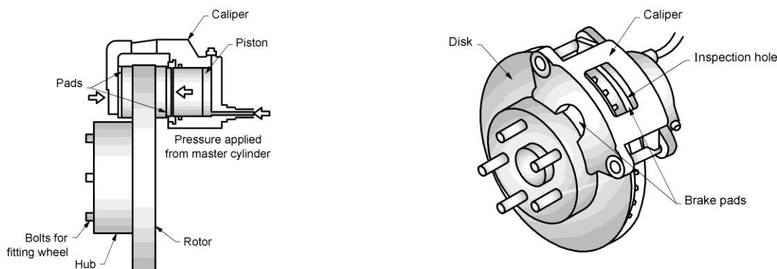
Fig. 7.15 Disc brake
